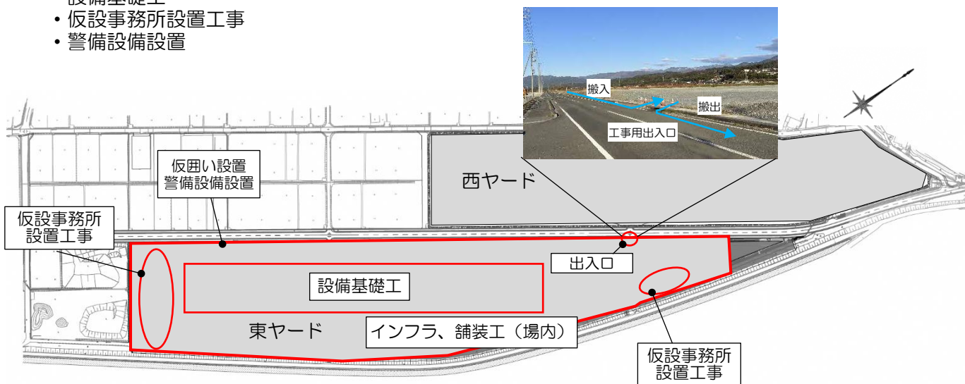
高森ヤード平面図
