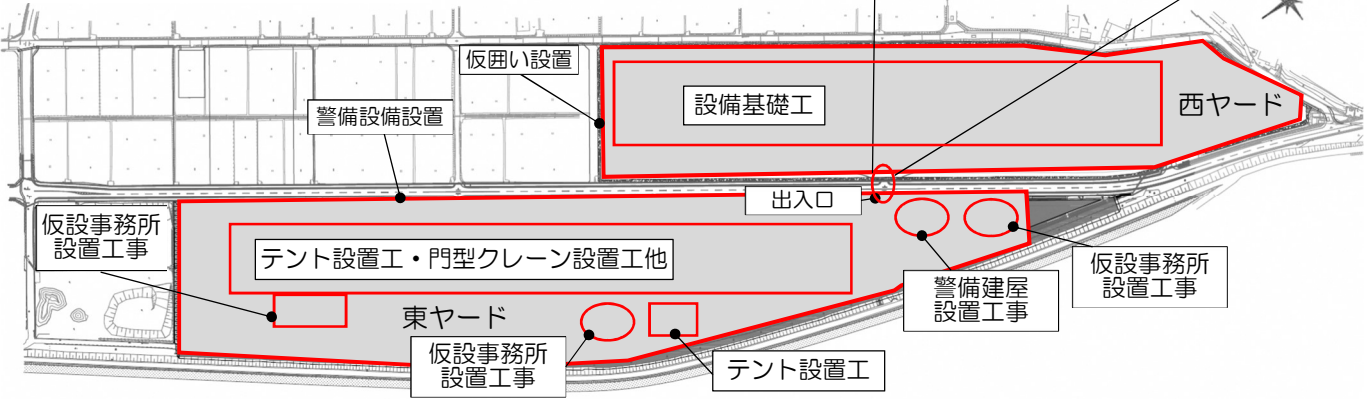
高森ヤード平面図
