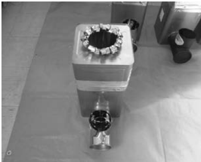
1 斗缶で作ったロケットストーブ
